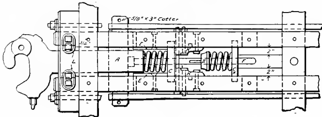
Fig. 1940. Plan.
